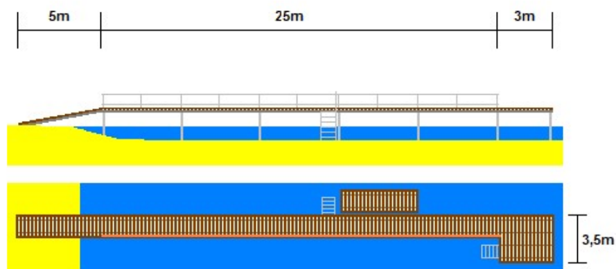
Figur 3: Principtegninger af broen.
